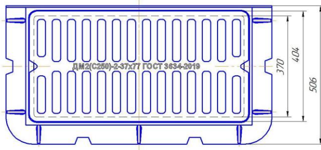
Материал корпуса и решетки - СЧ20 ГОСТ 1412-85
