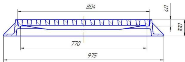
Дождеприемник ДМ2(С250)-2-37х77 ГОСТ 3634-2019
